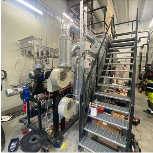
Installationer processbyggnad.
